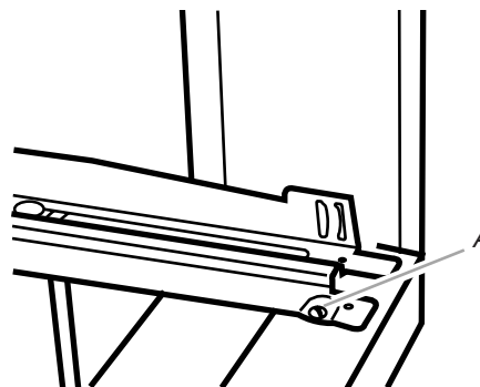
A. Tornillo para madera de cabeza ranurada #10 - 12 x 1½"
