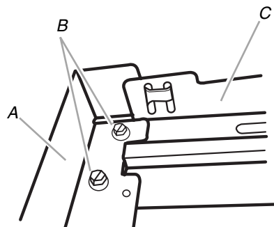
A. Barra posterior de la bandeja B. Tornillos de cabeza hexagonal #8 - 18 \times \frac{1}{4} " C. Barra lateral de la bandeja
