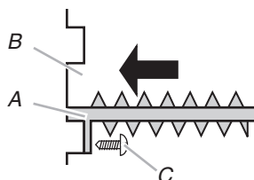
A. Cortina lateral contra la ranura de la ventana B. Ranura de la ventana C. Tornillo de cabeza redonda #8 x \frac{3}{4} "
