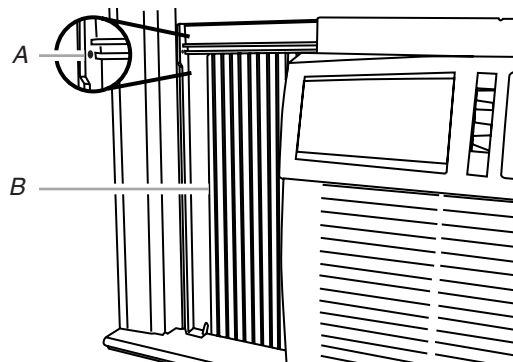
A. Orificio para el tornillo de cabeza redonda #8 x \frac{3}{4} " B. Cortina lateral
