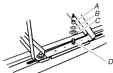
A. Tuerca hexagonal B. Arandela de presión C. Arandela plana D. Perno de carruaje
